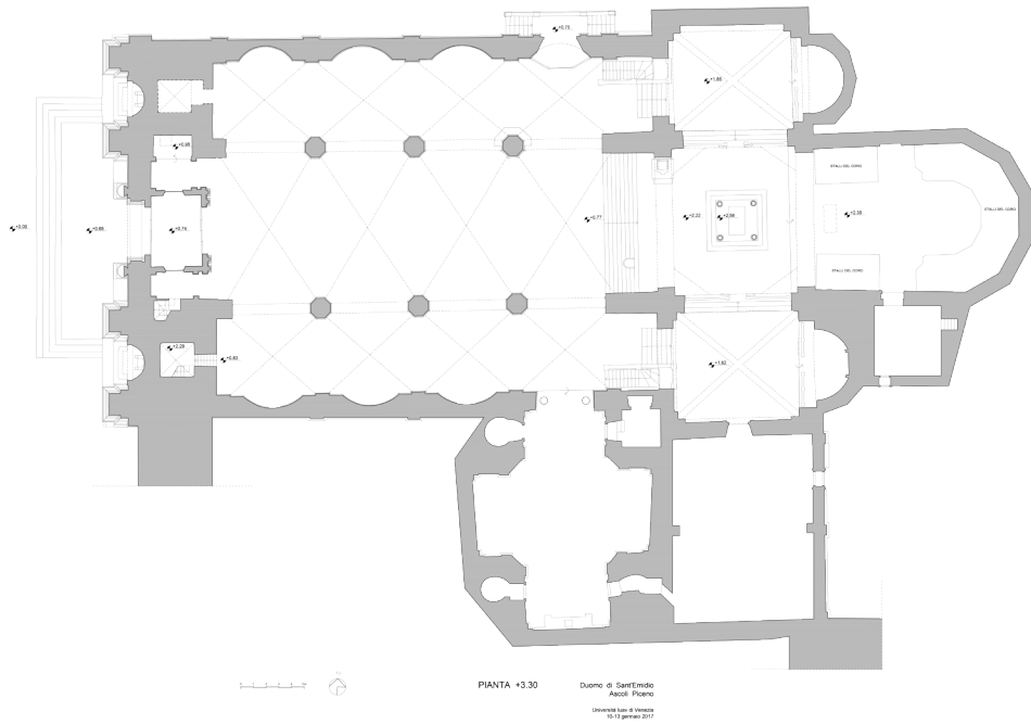
Fig. 15. Pianta del Duomo di Ascoli Piceno
